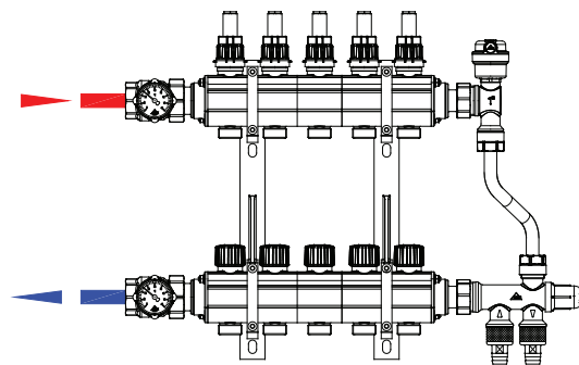
Corretta installazione del collettore con flussometro
